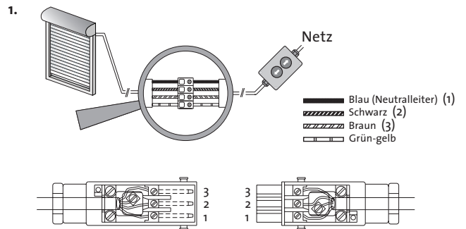
Stecker einführen
